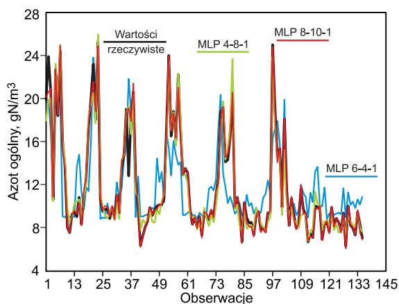
Rys. 3. Porównanie rzeczywistej zawartości azotu ogólnego w ściekach oczyszczonych oraz wartości prognozowanych za pomocą sztucznych sieci neuronowych
