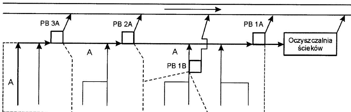
Rys. 1. Schemat sieci kanalizacyjnej do przykładu 2
