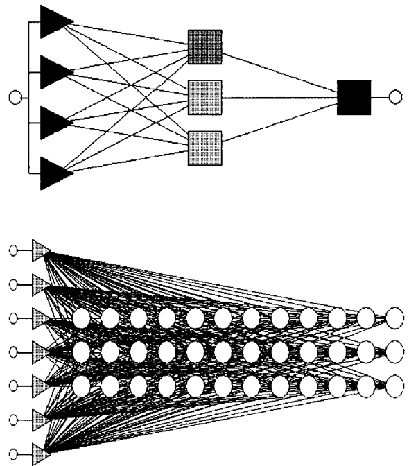
Rys. 2. Struktura sieci perceptronnej o pojedynczej warstwie ukrytej typu MLP s4 1:4-3-1:1 (góra) oraz sieci samoorganizującej Kohonena typu SOFM 7:7-36:1 (dół)
