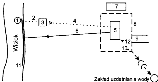
Rys. 2. Schemat stacji osłonowej wodociągu rzeszowskiego w Zarzeczcu
