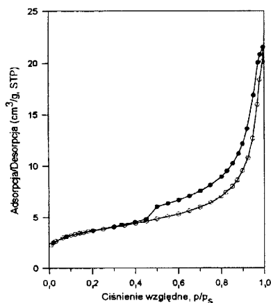
Rys. 1. Izoterma adsorpcji-desorpcji azotu na naturalnym klinoptylolicie
