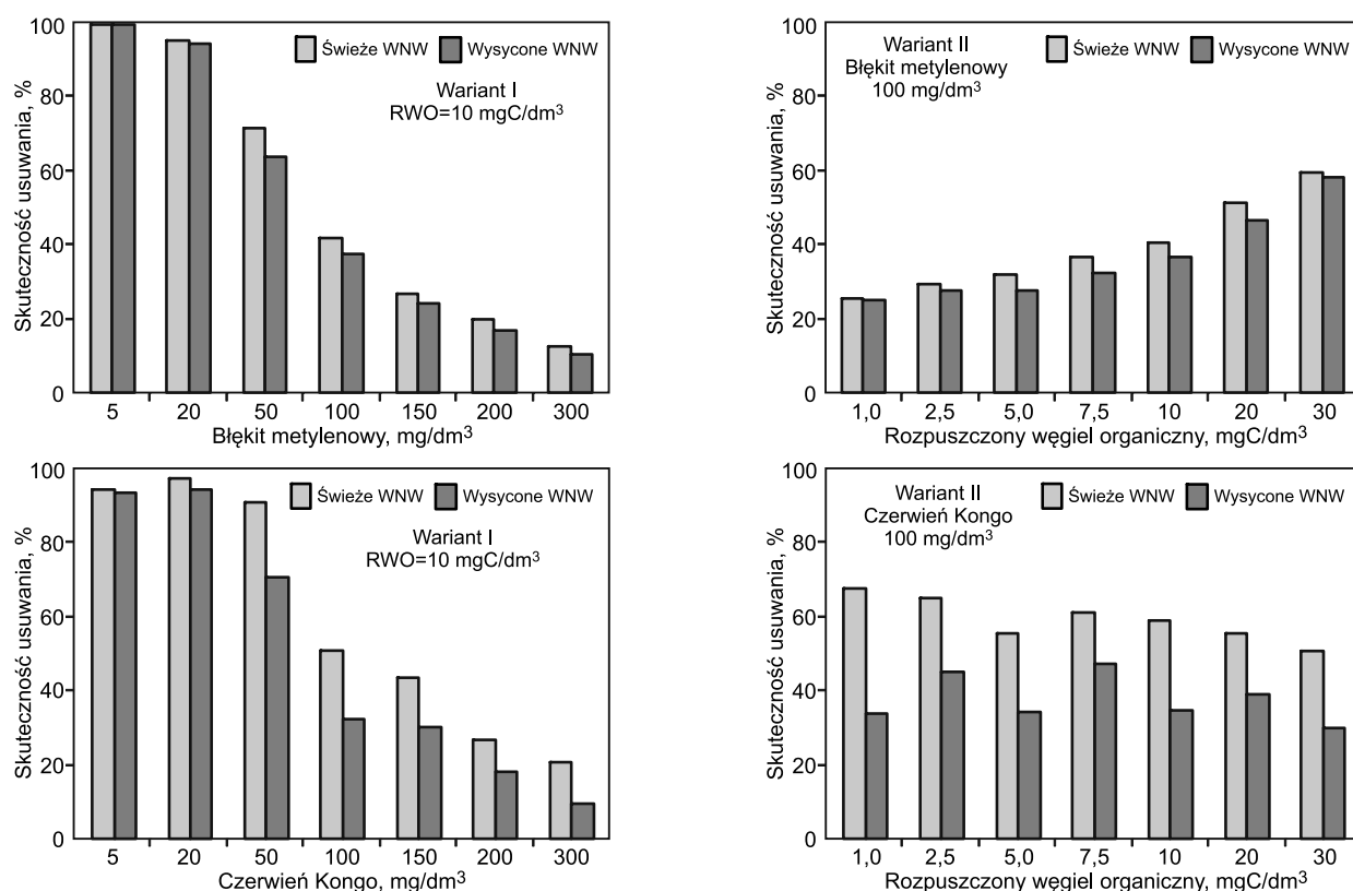
Rys. 4. Skuteczność usuwania błękitu metylenowego i czerwieni Kongo na świeżych i częściowo wysyconych nanorurkach węglowych z roztworów zawierających substancje humusowe
