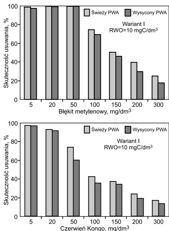
Rys. 3. Skuteczność usuwania błękitu metylenowego i czerwieni Kongo na świeżym i częściowo wysyconym pyłowym węglu aktywnym z roztworów zawierających substancje humusowe
