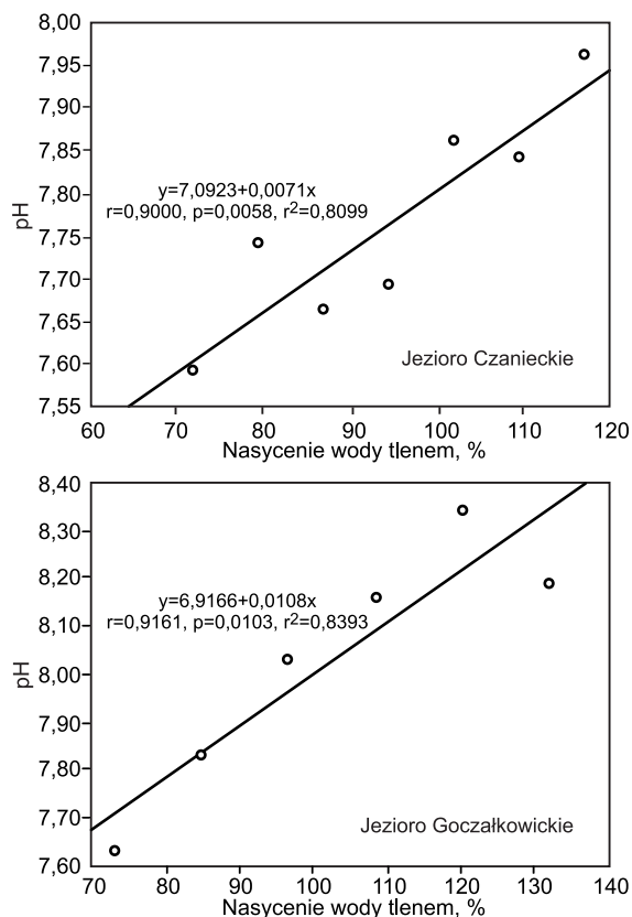
Rys. 9. Korelacja między wartością pH i stopniem nasycenia tlenem wody w Jeziorze Czańckim i Jeziorze Goczałkowickim
