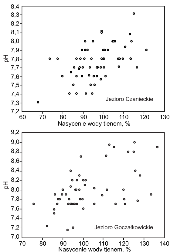
Rys. 8. Rozrzut wartości pH i stopnia nasycenia tlenem wody w Jeziorze Czańckim i Jeziorze Goczałkowickim
