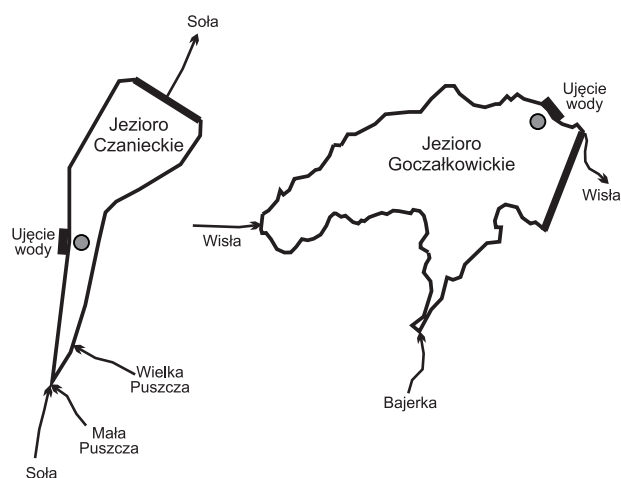
Rys. 1. Zarys zbiorników zaporowych wraz z lokalizacją punktów pomiarowo-kontrolnych w rejonie ujść wody
