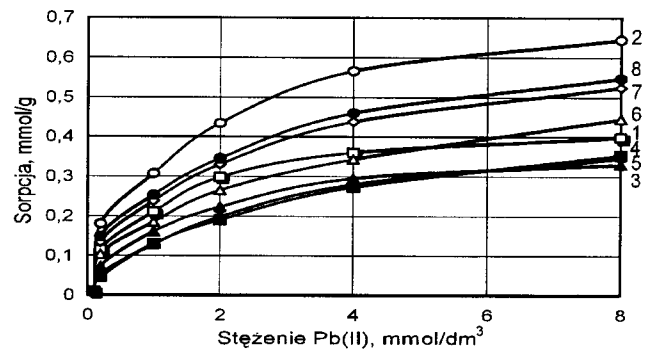
Rys. 5. Izoterm sorpcji jonów Pb(II) na węglach A2PS-1+A2PS-8
