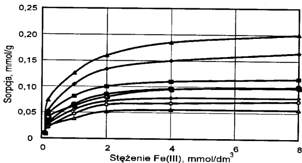
Rys. 4. Izoterm sorpcji jonów Fe(III) na węglach A2PS-1+A2PS-8
