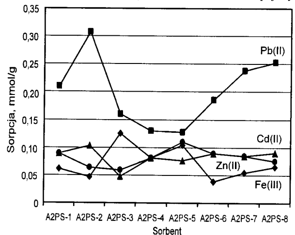
Rys. 7. Porównanie sorpcji jonów metali przy stałym stężeniu roztworu ( 1 \text{ mmol/dm}^3 ) na węglach A2PS-1+A2PS-8
