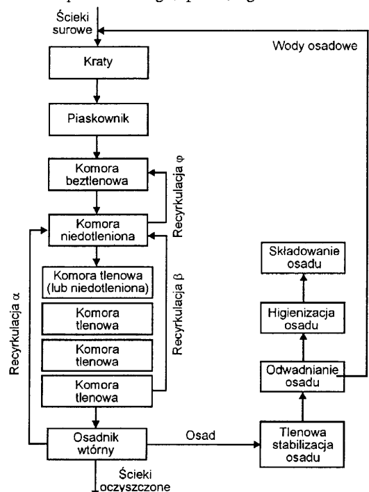
Rys. 2. Schemat technologiczny oczyszczalni ścieków w Kartuzach
