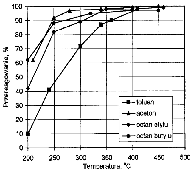
Rys. 1. Skuteczność przereagowania wybranych związków organicznych na katalizatorze PER-1
