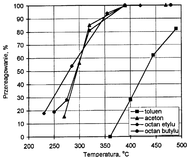
Rys. 3. Skuteczność przereagowania wybranych związków organicznych na katalizatorze TE-1
